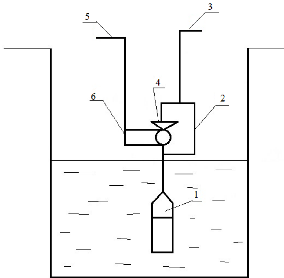
Рис. 3. Схема насосной установки со струйным насосом:
