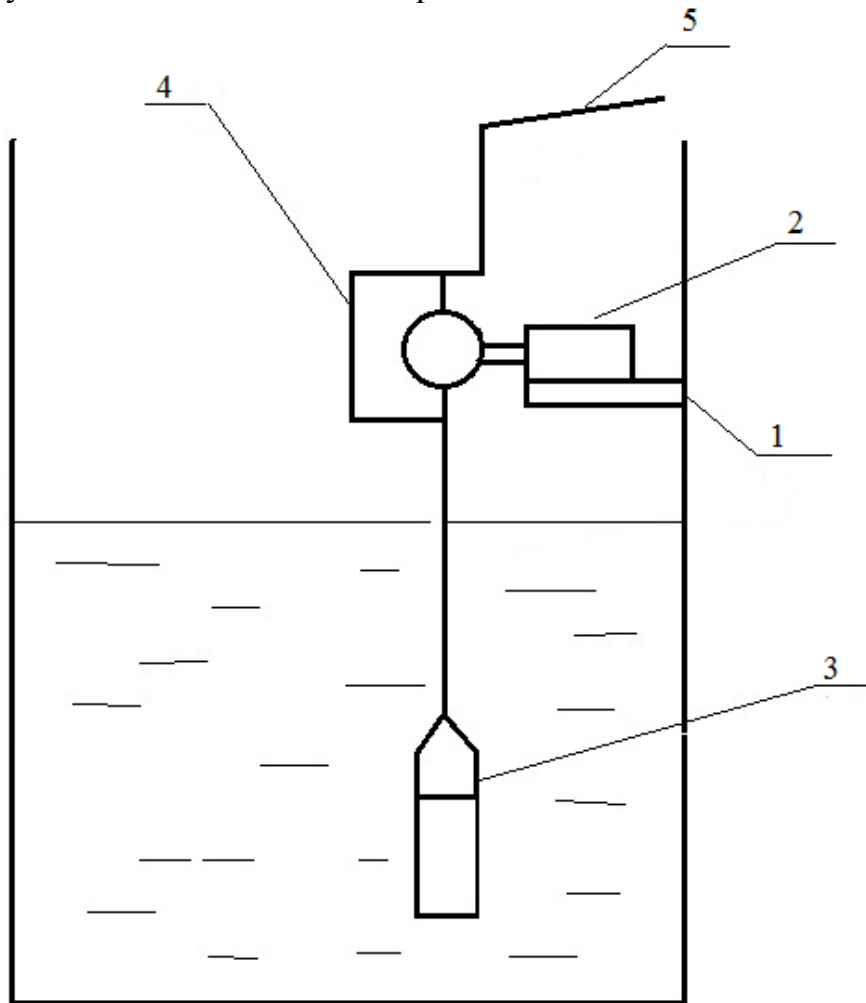
Рис. 1. Схема насосной установки с дополнительным электронасосом: 1 – полок; 2 – дополнительный электронасос; 3 – основной электронасос; 4 – обводной трубопровод; 5 – напорный трубопровод.
